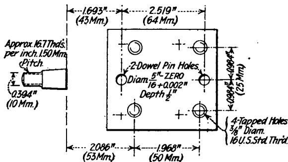
FIG. 56.—Magneto base.
