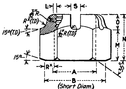
FIG. 55.—Plain castle nut.
